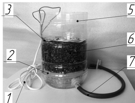
Рисунок 2. Модель экспериментальной установки: 1-кабель питания; 2- пластина графитовая; 3- пластина алюминиевая; 5- сосуд; 6- кальцит силицированный; 7- патрубок слива готовой воды
