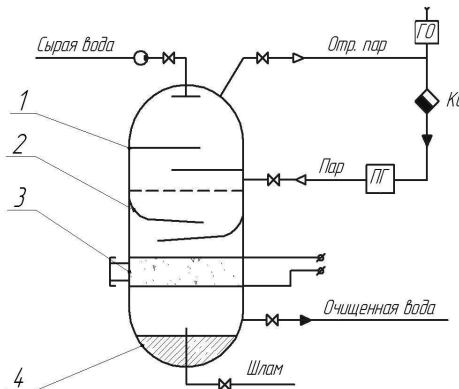
Рисунок 1. Схема модернизированной мобильной системы
